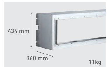
Fan Casing
