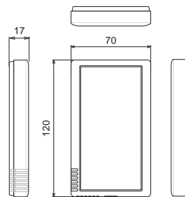
REMOTE SENSOR (CZ-CSRC3)
